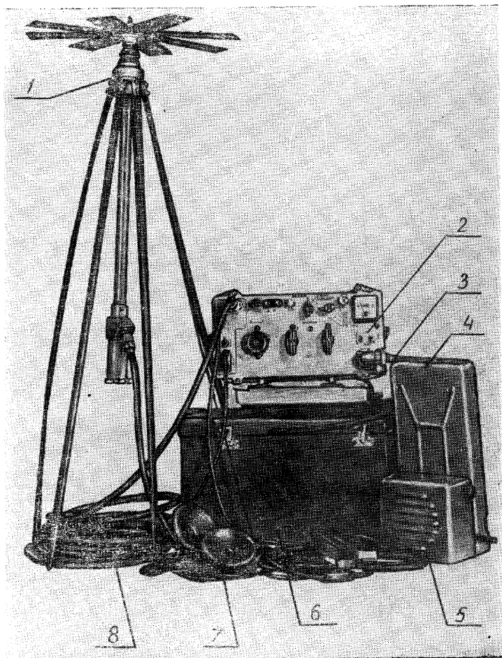
Рис. 1.1. Общий вид радиоприемника.
